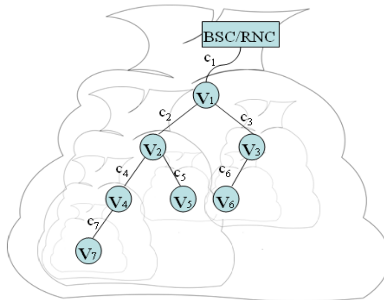
圖 11、CCN-BA 巢狀背包問題
