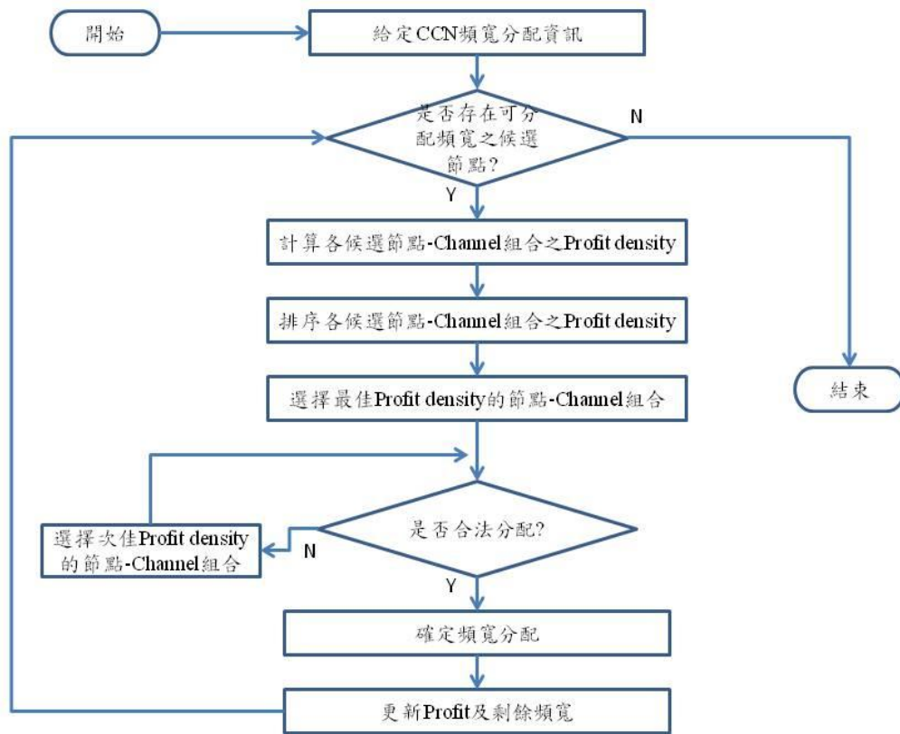
圖 12、BAG 演算法流程
