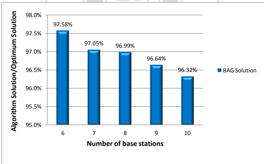
圖 28、實驗二基地台數量與效能之關係-平均最佳解達成率
