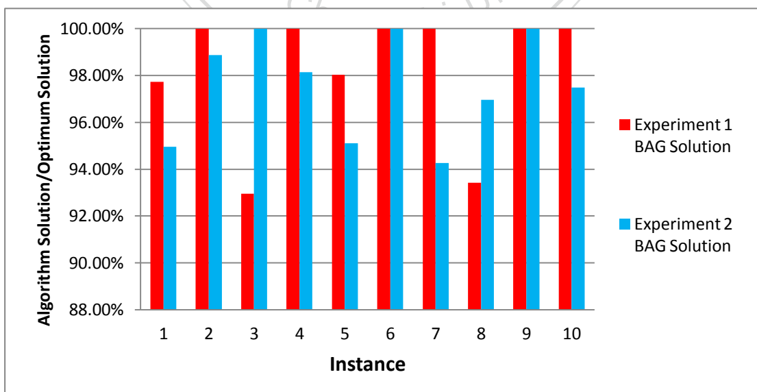
圖 33、BAG 演算法效能比較(6 個基地台)
