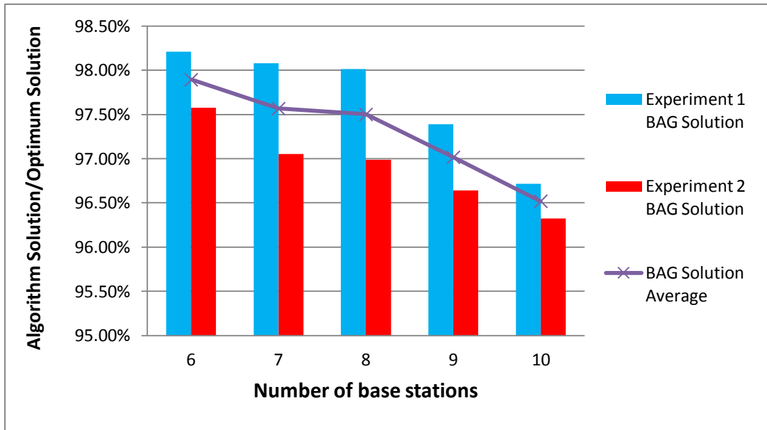
圖 32、基地台數量與效能之綜合評估-平均最佳解達成率
