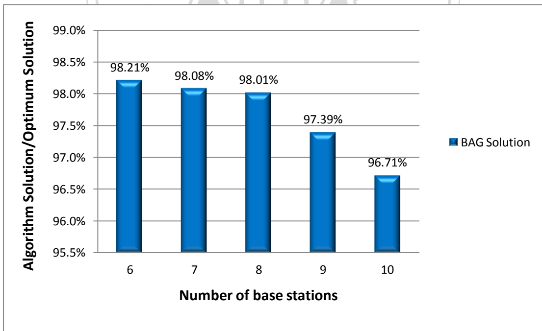
圖 26、實驗一基地台數量與效能之關係-平均最佳解達成率
