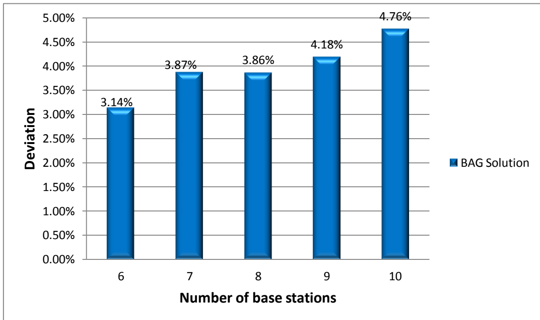
圖 27、實驗二基地台數量與效能之關係-平均誤差
