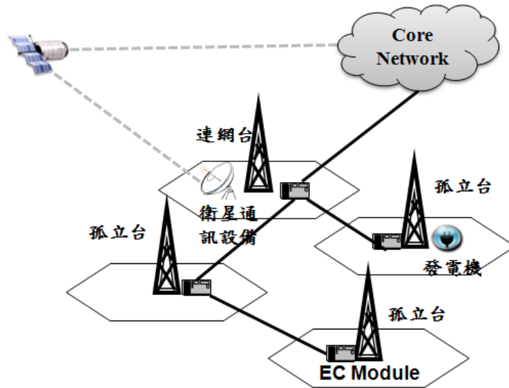
圖 8、CCN 網路架構圖
