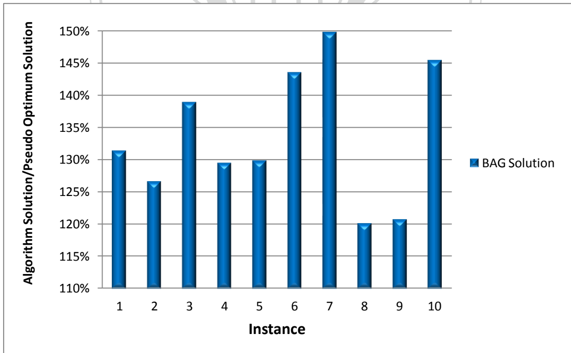
圖 30、大規模系統下 BAG 演算法效能-準最佳解達成率(100 個基地台)
