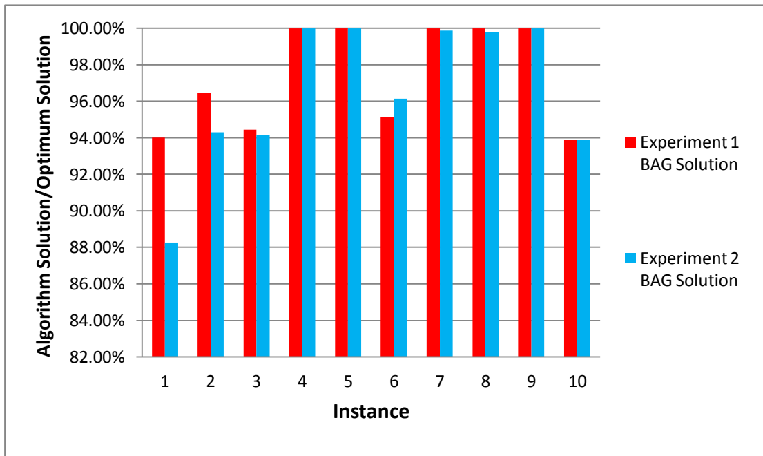
圖 36、BAG 演算法效能比較(9 個基地台)
