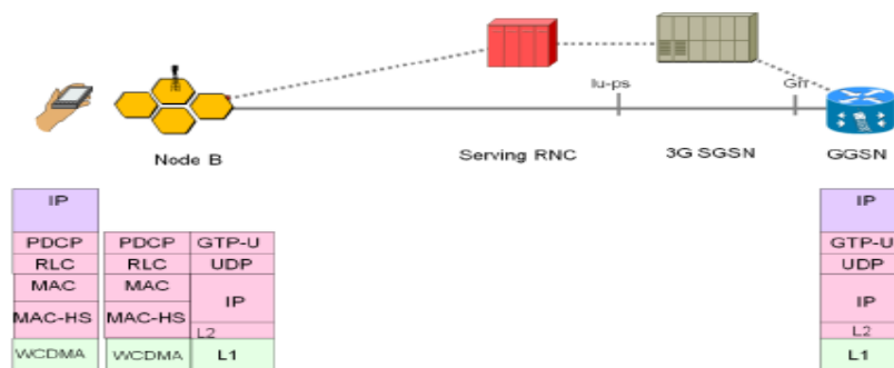
圖 7、3GPP Release 7 架構
