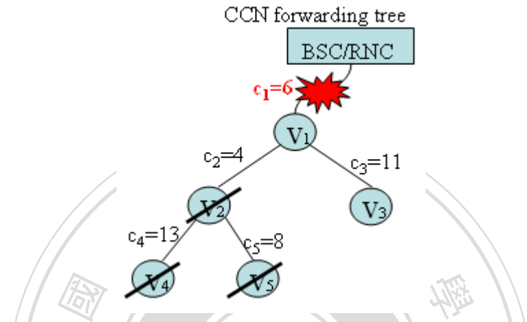
圖 22、範例-時間點四之候選節點
