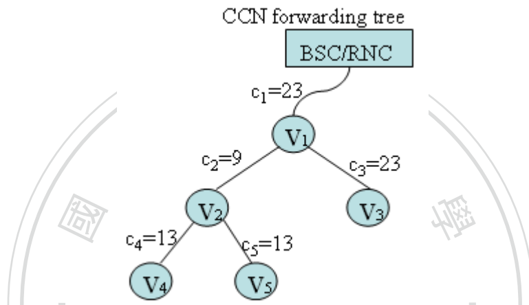
圖 17、範例-時間點一頻寬分配後樹狀轉送拓樸剩餘頻寬
