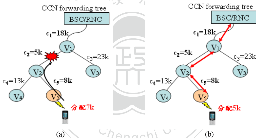
圖 14、範例-CCN traffic relay 及頻寬限制
