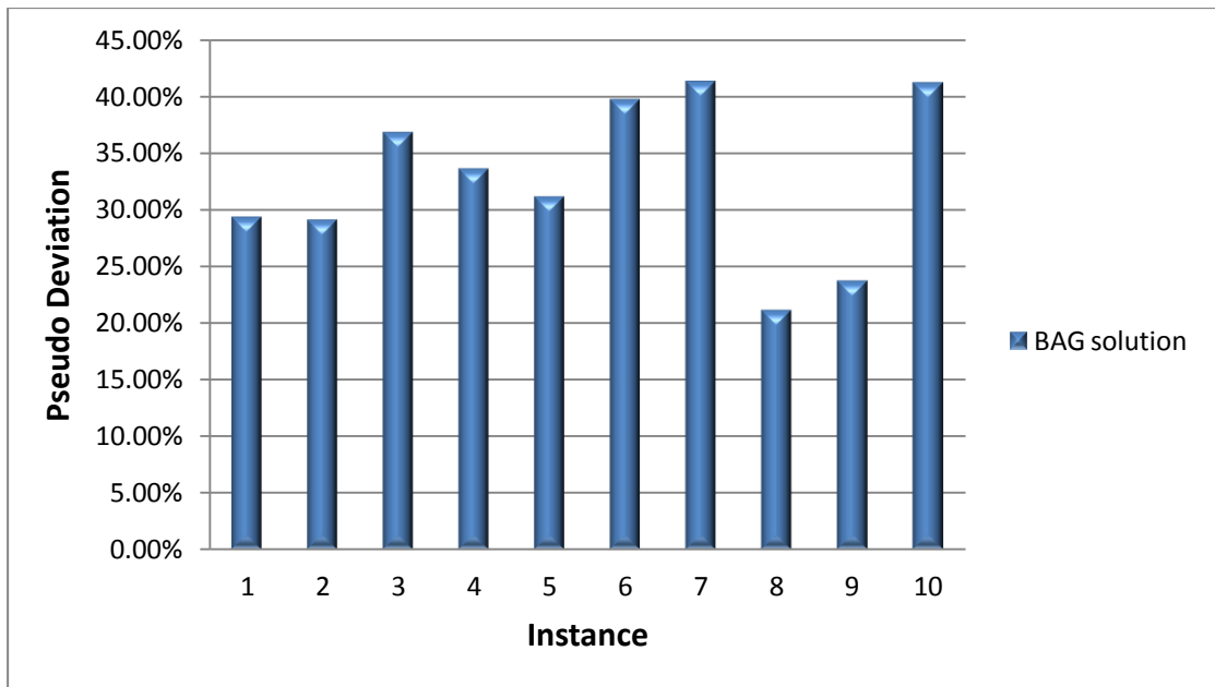
圖 29、大規模系統下 BAG 演算法效能-準誤差(100 個基地台)
