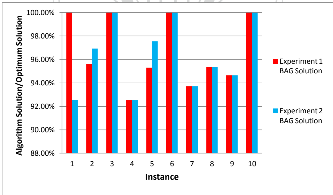
圖 37、BAG 演算法效能比較(10 個基地台)
