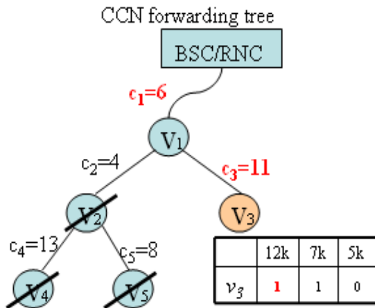
圖 21、範例-時間點三頻寬分配後樹狀轉送拓樸剩餘頻寬
