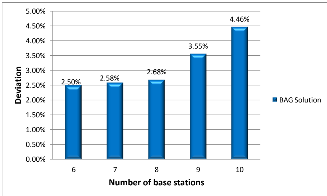
圖 25、實驗一基地台數量與效能之關係-平均誤差
