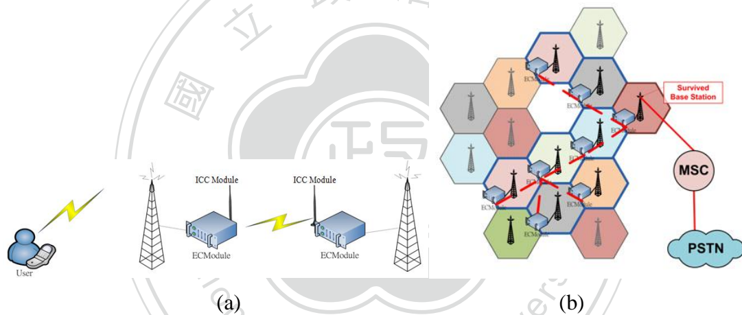
圖 10、孤立台恢復連線方式
