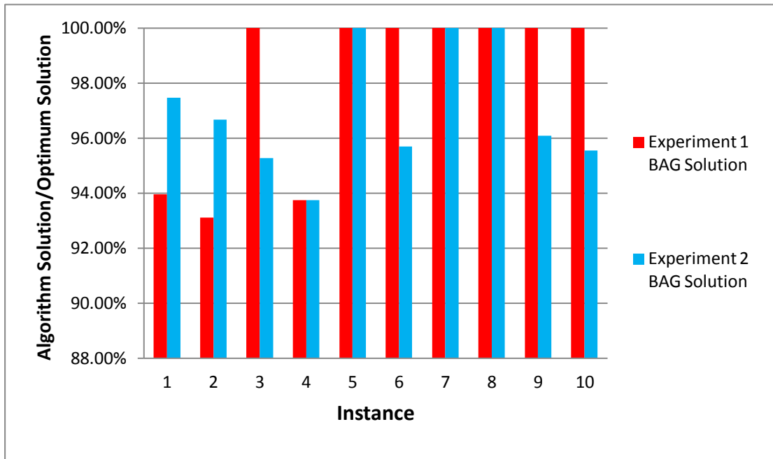
圖 34、BAG 演算法效能比較(7 個基地台)
