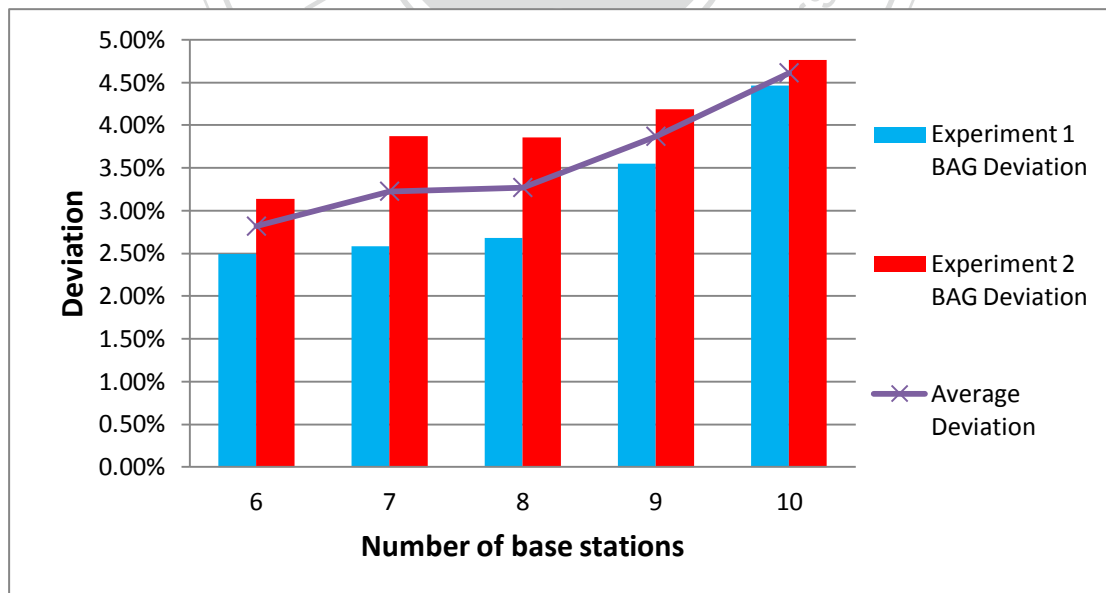
圖 31、基地台數量與效能之綜合評估-平均誤差
