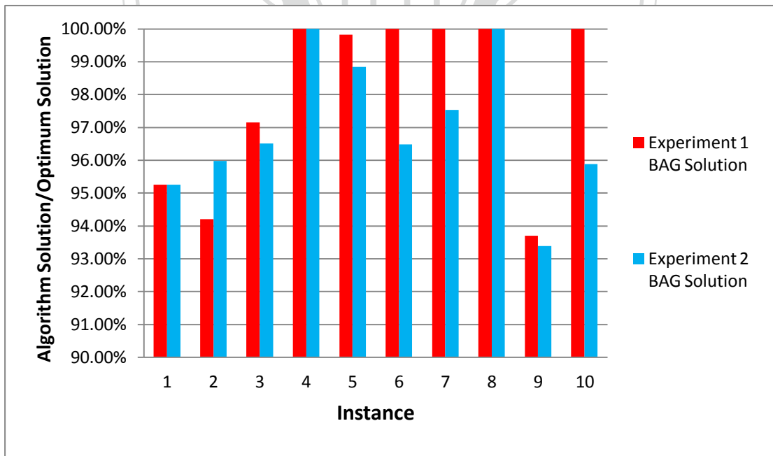
圖 35、BAG 演算法效能比較(8 個基地台)
